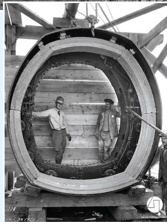
Μηχανικός και εργάτης του έργου φωτογραφίζονται στον μεγάλο μεταλλικό δακτύλιο που χρησιμοποιήθηκε για την κατασκευή της Σήραγγας του Μπογιατίου, 1928. Πηγή: Ιστορικό Αρχείο ΕΥΔΑΠ
